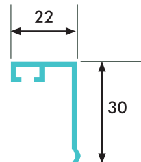
Standart Çerçeve Standard frame
