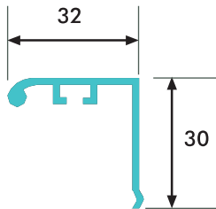
Dar Çerçeve Narrow frame
