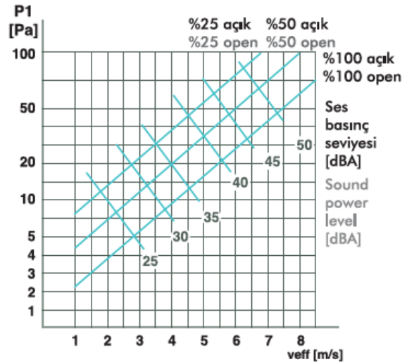
Zıt kanatlı damperli kare petek menfez basınç kaybı ve ses seviyeleri. Egg crate grille with opposed blade damper pressure loss and sound power levels.
