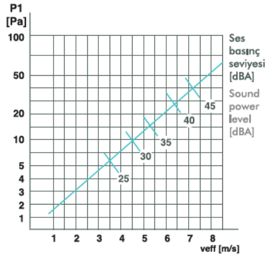
Kare petek menfez basınç kaybı ve ses seviyeleri. Return grille pressure loss and sound power levels.
